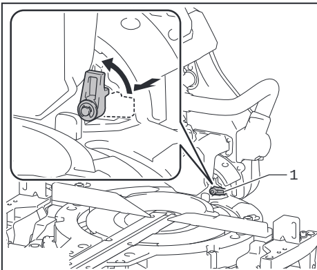
► 1. Latch lever
