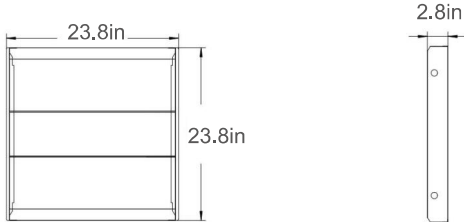
2X2 Troffer
