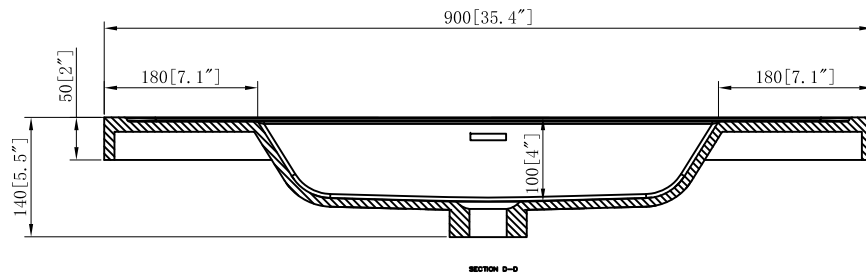
SECTION D-D
