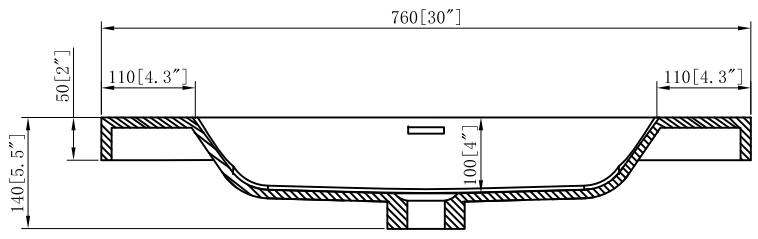
SECTION D-D
